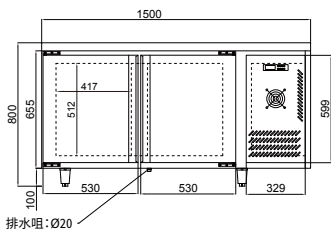
正面圖 Front View
