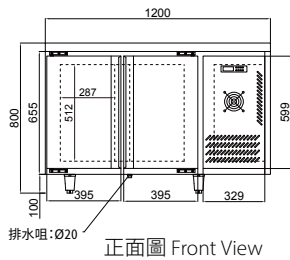
正面圖 Front View
