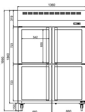
正面圖 Front View
