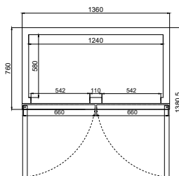
俯視圖 Top View
