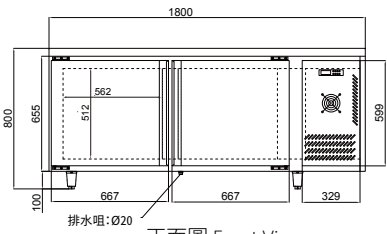
正面圖 Front View
