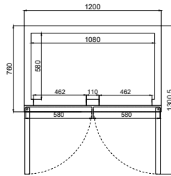
俯視圖 Top View
