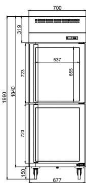
正面圖 Front View
