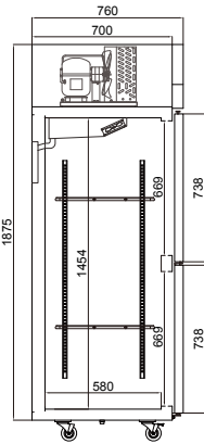
側視圖 Profile Plane
