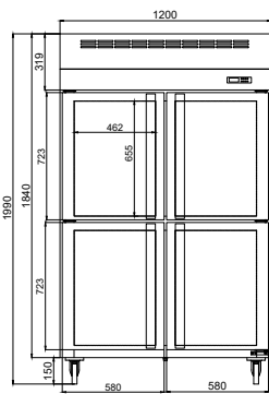
正面圖 Front View
