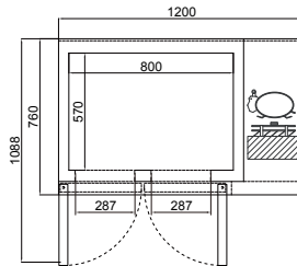
俯視圖 Top View
