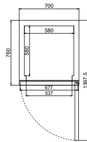
俯視圖 Top View
