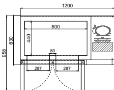
俯視圖 Top View
