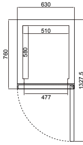
俯視圖 Top View
