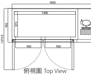
俯視圖 Top View
