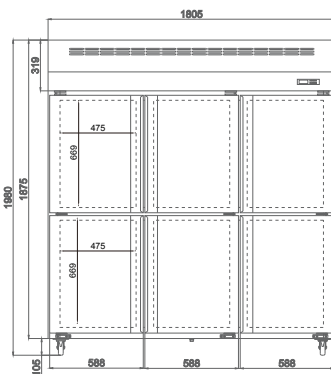
正面圖 Front View
