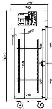
側視圖 Profile Plane
