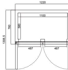
俯視圖 Top View
