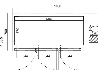
俯視圖 Top View
