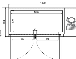
俯視圖 Top View
