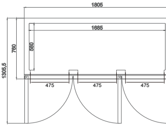
俯視圖 Top View
