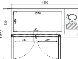
俯視圖 Top View
