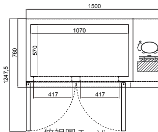
俯視圖 Top View
