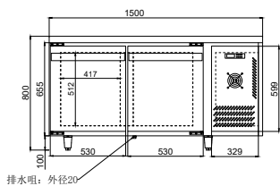
正面圖 Front View
