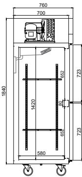
側視圖 Profile Plane
