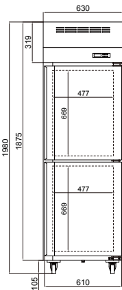
正面圖 Front View
