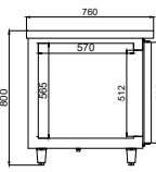
側視圖 Profile Plane
