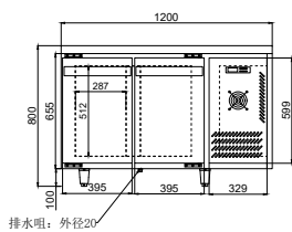
正面圖 Front View
