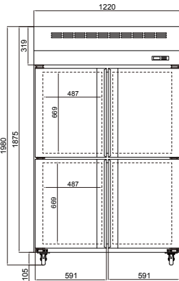
正面圖 Front View
