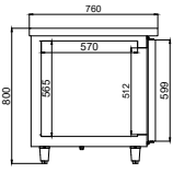
側視圖 Profile Plane
