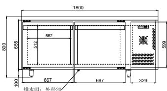
正面圖 Front View
